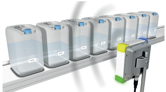
Marquage personnalisé du produit individuel et saisie simultanée de plusieurs supports de données avec RFID UHF
